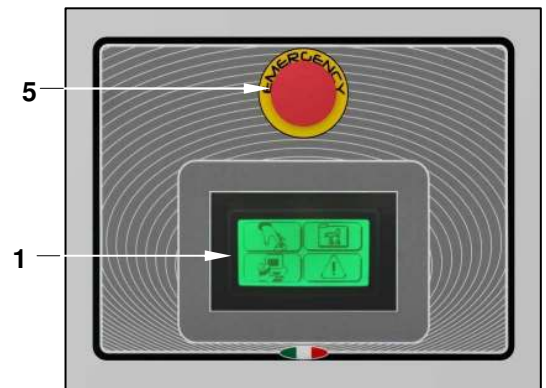
Рисунок 4 – Панель управления версий PL120 и PL140 с ПЛК мод. NVAP
