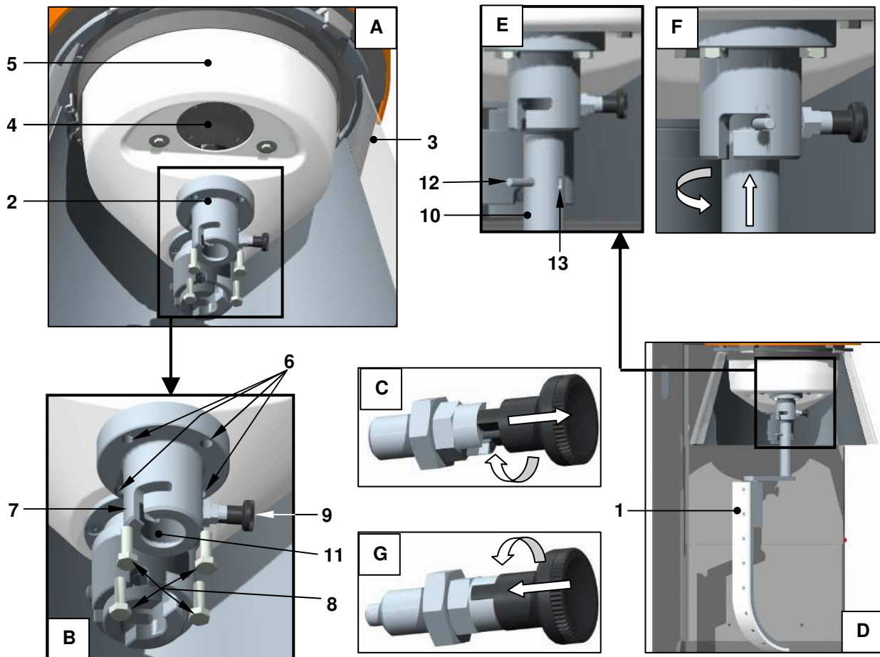
Рисунок 12– Установка/извлечение скребка
