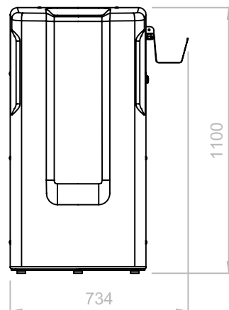
СБОКУ
