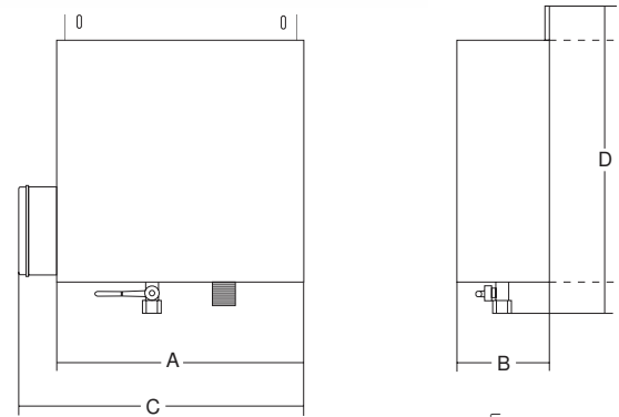
STERILIZZATORE ELETTRICO
