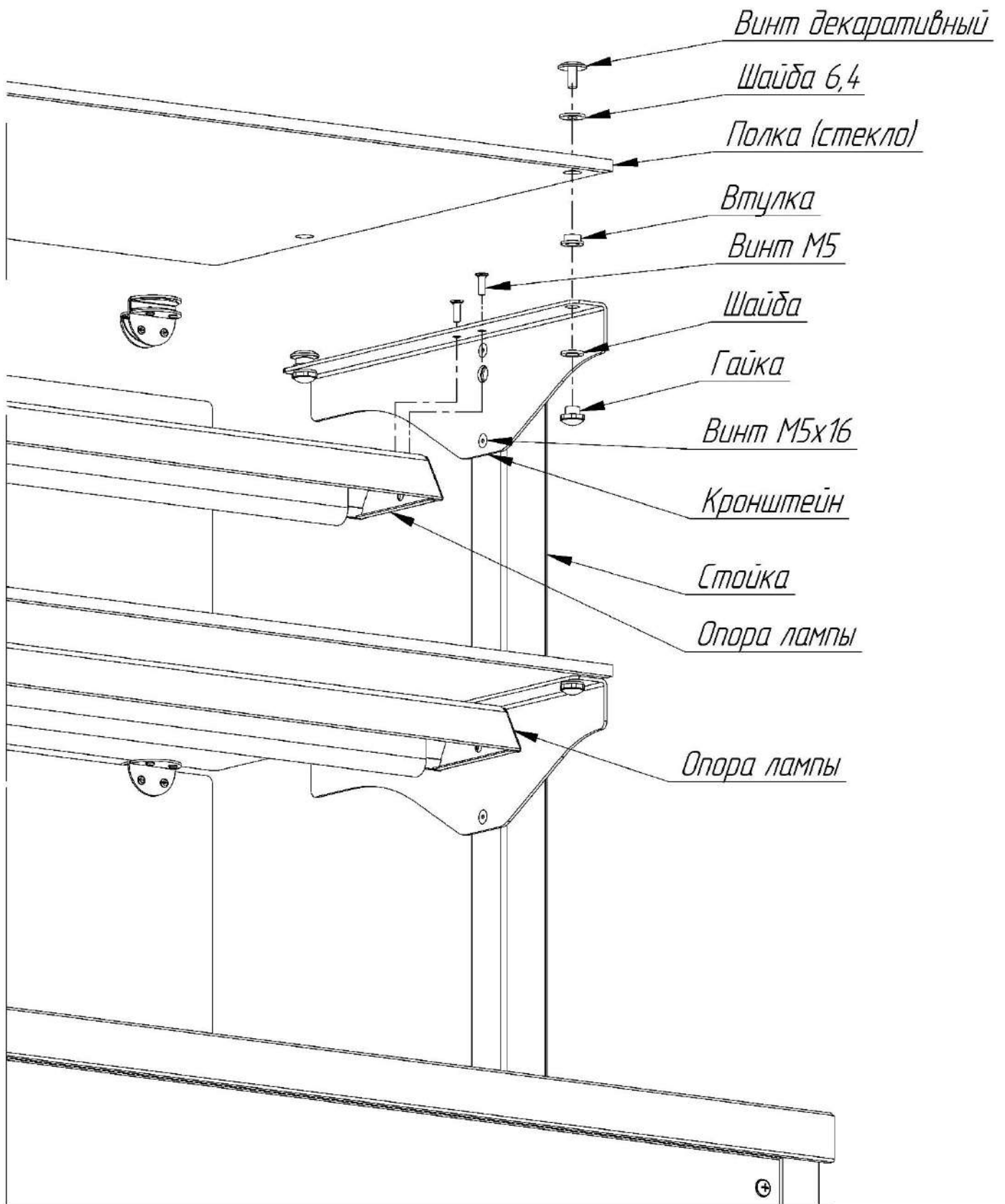
Рис.2 Сборка полок.
